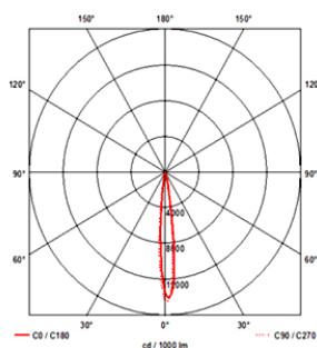
NAMIB 80 L 12°
