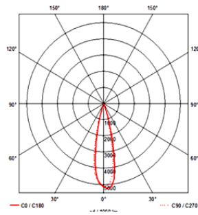
NAMIB 80 L 24°
