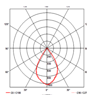
NAMIB80 L 60°
