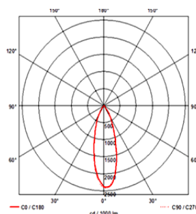
NAMIB 80 L 33°
